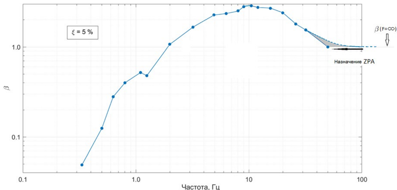
Рисунок А.1 – Схема назначения частоты, соответствующей УНП (спектр реакции для воздействия с единичным пиковым ускорением)
