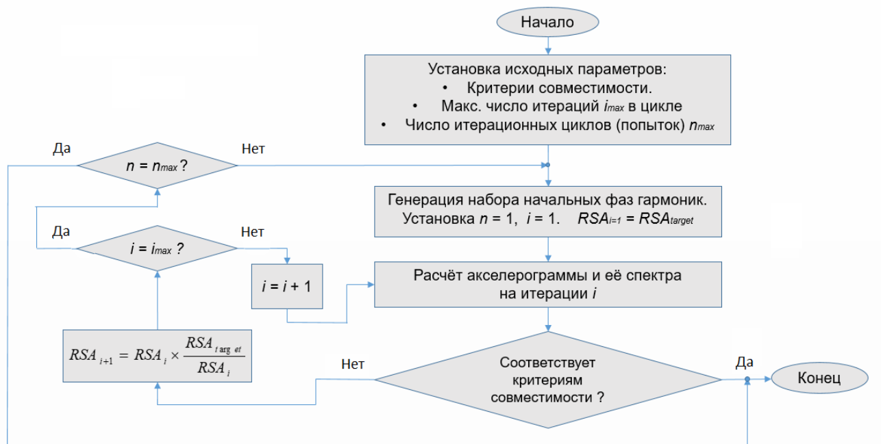
Рисунок 15.4.1.1 – Алгоритм расчёта синтетической акселерограммы
