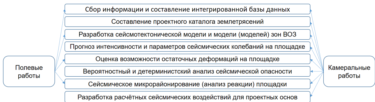
Рисунок 5.1 – Блок-схема работ по ОСО и РСВ
