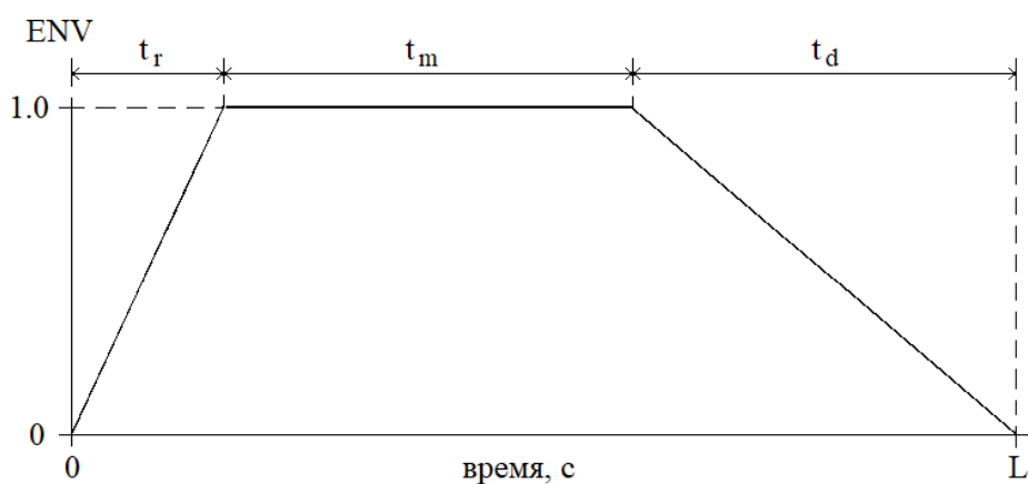
Рисунок В.1 – Форма огибающей обобщённой синтезированной акселерограммы
